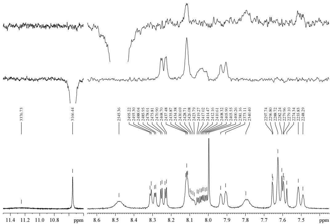
87. ábra. VIC31772 vegyület, RG1475T minta ^1\text{H} -NMR spektrumának Gauss ablakfüggvénnyel (LB = -1, GB = 0.25) javított felbontású részlete, valamint a minta két szelektív 1D zqs-easy ROESY felvétele. 2 * 100 msec keverési idő randomizálás nélkül, 128 scan.
