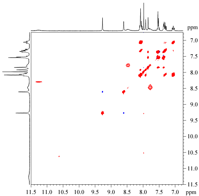
97. ábra. VIC31874 vegyület, RG1505 minta zqS-TOCSY spektruma; 2 scan * 192 kísérlet, \tau_{\text{mix}} = 70 msec
