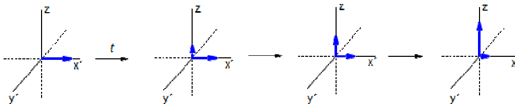
30. ábra. A longitudinális T_1 relaxáció mechanizmusa. Az xy síkban megszűnő mágnesezettséggel azonos eredő mágnesezettség épül ki a z tengely irányában. Az ábra forrása ref. [78]
