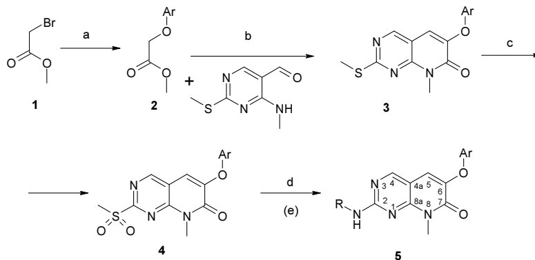
112. ábra. 6-ariloxi-2-(alkilamino)-8-methyl-8H-pirido[2,3-d]pirimidin-7-on származékok előállítása.
