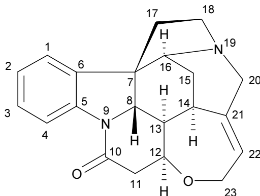
39. ábra. A modellvegyületként használt sztrichnin szerkezete és vázatomjainak számozása. (összegképlete: C_{21}H_{22}N_2O_3 , relatív molekulatömeg: 334.42).
