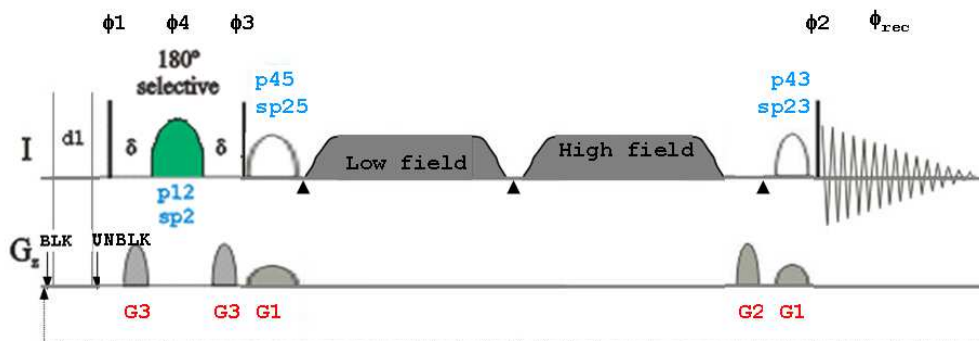
54. ábra. A spfge-se offszet-kompensált zéró-kvantum elnyomós adiabatikus szelektív 1D ROESY (spfge-se-1D-zqs-easy-ROESY) folyamatábrája.
