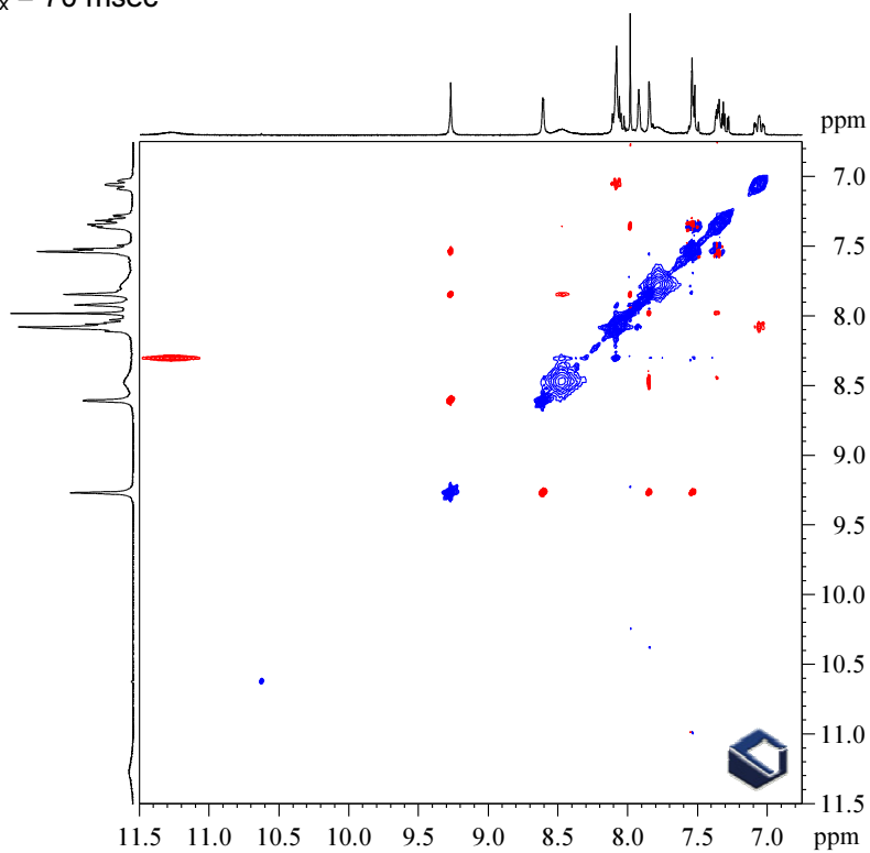
98. ábra. VIC31874 vegyület, RG1505 minta zqS-easy-random ROESY spektruma; 8 scan * 192 kísérlet, \tau_{\text{mix}} = 2 * 100 ms \pm 5 %, \theta = 54.7^\circ , lineáris predikció és zéró töltés után digitális felbontás, 1.5 Hz/pont.
