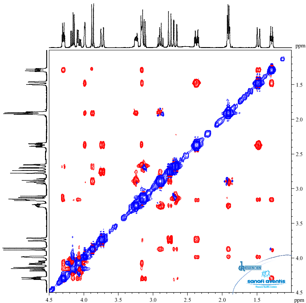
43. ábra. A sztrichnin offszet-kompenzált, zéró-kvantum elnyomásos (zqs-easy-) ROESY spektruma [IV]
