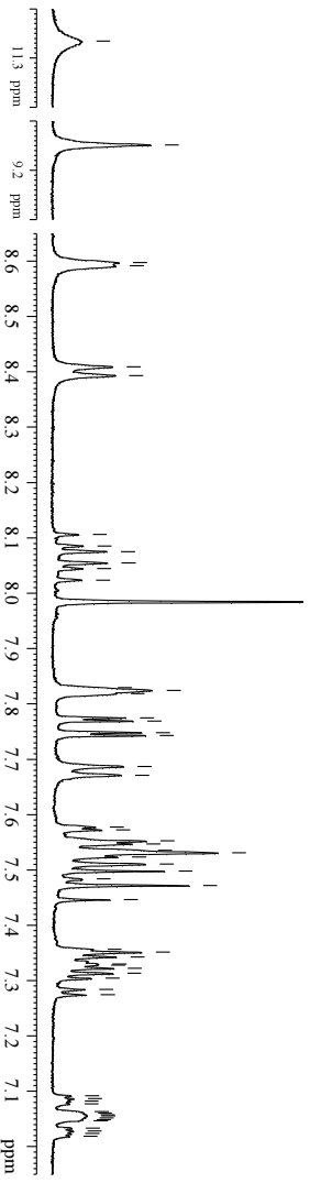
105. ábra. VIC31872 vegyület, RG1503 minta ^1\text{H-NMR} spektruma Gauss ablakfüggvénnyel (LB = -1, GB = 0.25) javított felfontású részlet spektruma; a spektrum fölött a csúcslista Hz mértékegységben. A spektrum fölött három különböző szelektív 1D zqs-TOCSY spektrum, minden TOCSY spektrum fölött feltüntetve a kiválasztott jel és az alkalmazott optimalizált keverési idő.
