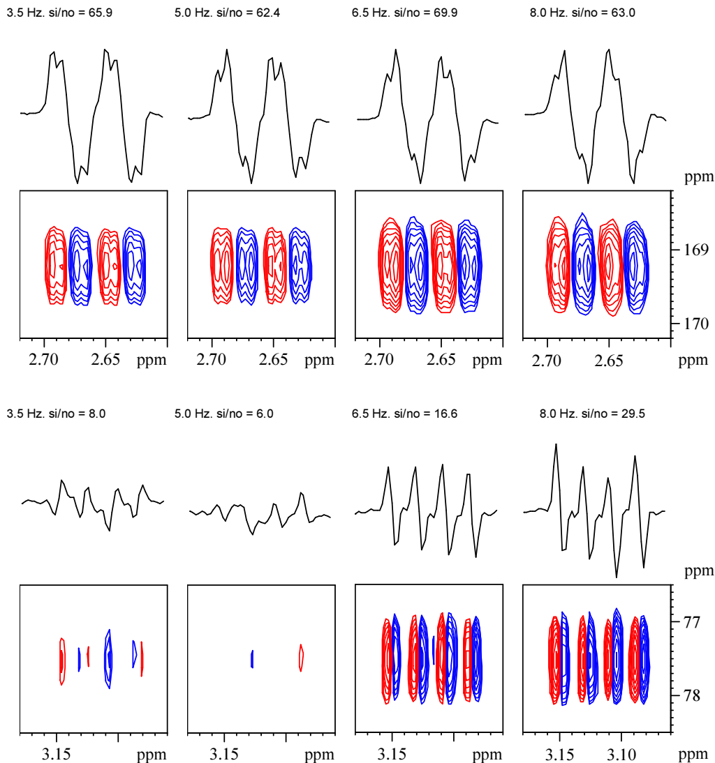
6. ábra. Két kiválasztott jel jelalakjának és jel/zaj viszonyának függése a csatolási állandónak a mérés paraméterezése során beállított optimumától.
