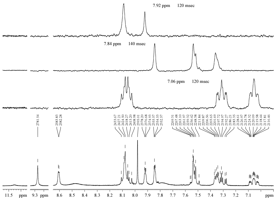
96. ábra. VIC31874 vegyület, RG1505 minta ^1\text{H-NMR} spektrumának Gauss ablakfüggvénnyel (LB = -1, GB = 0.25) javított felbontású részlete, a spektrum fölött Hz listával. A spektrum fölött három különböző szelektív 1D zqs-TOCSY spektrum, minden TOCSY spektrum fölött feltüntetve a kiválasztott jel és az alkalmazott optimalizált keverési idő.
