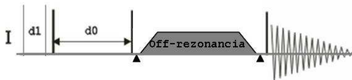
36. ábra. Az off-rezonancia ROESY módszerváltozat [86] folyamatábrája
