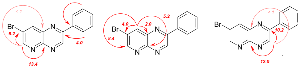
13. ábra. A KS0583VR minta – pirido-pirazin származék - spektrumainak értékelése, ^1\text{H} - és ^{13}\text{C} -NMR jelhozzárendelés, valamint a heteronukleáris távolható csatolási állandók értelmezése.
