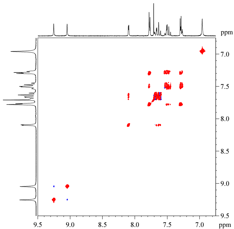
82. ábra. VIC31359 vegyület, RG1352 minta zqs-TOCSY spektruma; 2 scan * 192 kísérlet, T_{mix} = 70 msec
