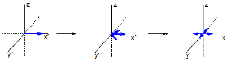
31. ábra. A transzverzális T_2 relaxáció mechanizmusa. A kezdetben koherens mágnesezettség az xy síkban szétszóródik, de nem kíséri mágnesezettség kiépülése a z tengely irányában. Az ábra forrása ref. [78]
