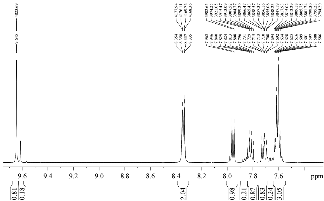
26. ábra. LA182X1 minta ^1\text{H} -NMR spektruma, az alsó csúcslista ppm dimenzióban a kémiai eltolódás pontos leolvashatósága miatt, a felső csúcslista pedig Hz dimenzióban, melyből a J(\text{H},\text{H}) és J(\text{F},\text{H}) csatolási állandók olvashatók le.
