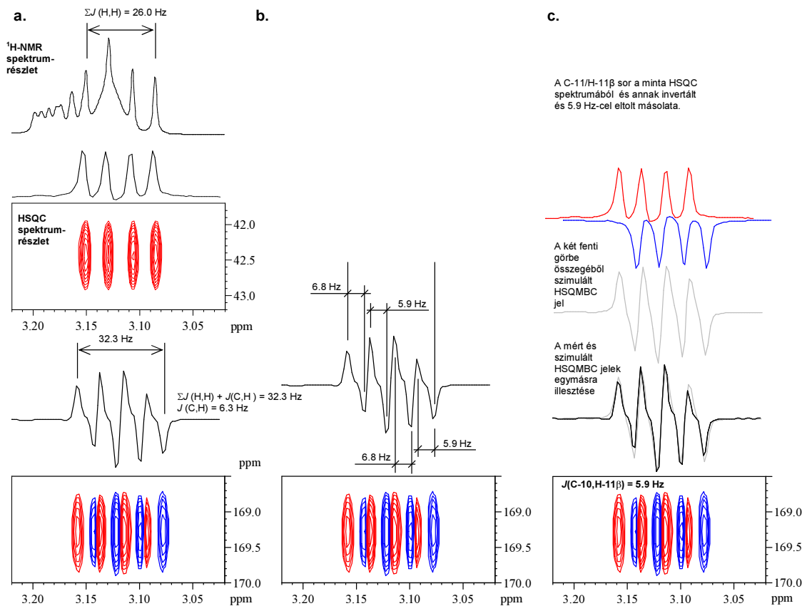
5. ábra. A keresett csatolási állandó kinyerésének lehetséges módszerei a HSQMBC spektrumból, a sztrichnin HSQMBC spektrumának C-10/H-11 \beta keresztcsúcsán demonstrálva.
