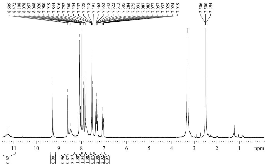
94. ábra. VIC31874 vegyület (17e sorszámú az V. számú saját publikációban), RG1505 minta átnézeti ^1\text{H} -NMR spektruma
