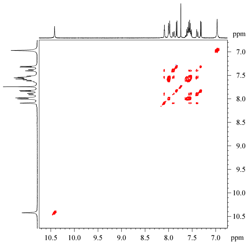
72. ábra. VIC31371 vegyület, RG1365 minta zqs-TOCSY spektruma, 2 scan * 192 kísérlet, \tau_{mix} = 70 msec.
