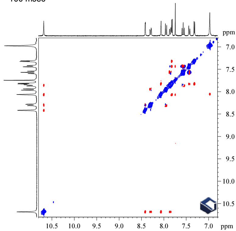
78. ábra. VIC31338 vegyület, RG1331 minta zqs-easy-random-ROESY spektruma, 8 scan * 128 kísérlet, T_{mix} = 2 * 100 msec \pm 5 %, \theta = 54.7^\circ , lineáris predikció és zéró töltés után digitális felbontás 1.4 Hz/pont. A ROESY spektrumban a 6.97/8.08 keresztcsúcs a víz betükröződése.
