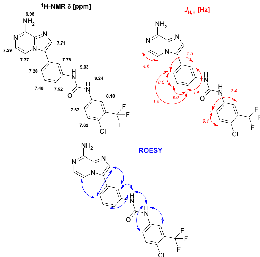
84. ábra. VIC31359 vegyület, RG1352 minta (16j sorszám az V. számú saját publikációban) 1 H-NMR, zqs-TOCSY és zqs-easy-random-ROESY spektrumainak értelmezése, jelhozzárendelésük.
