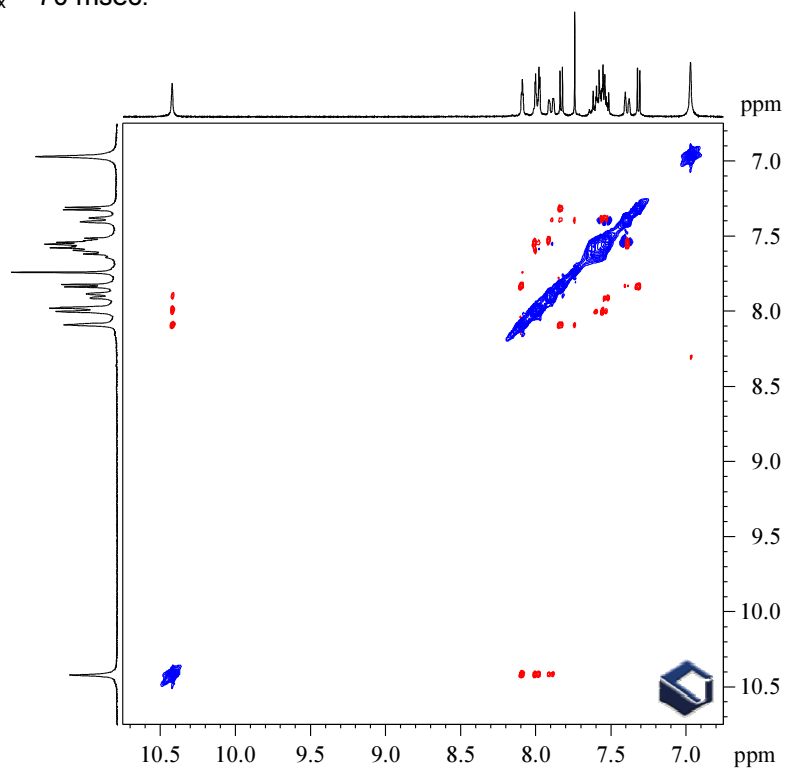
73. ábra. VIC31371 vegyület, RG1365 minta zqs-easy-random-ROESY spektruma, 8 scan * 192 kísérlet, \tau_{mix} = 2 * 100 msec \pm 5 %, \theta = 54.7^\circ , lineáris predikció és zéró töltés után digitális felbontás 1.5 Hz/pont.
