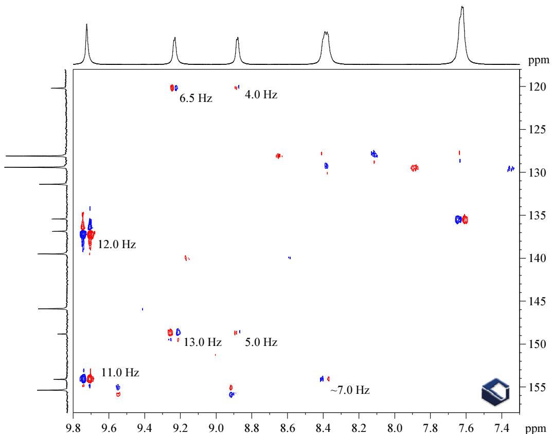
14. ábra. SZ12264A minta – pirido-pirazin származék - HSQMBC spektruma DMSO- d_6 oldószerben 30 °C-on. A leolvasott heteronukleáris csatolási állandók az ábrán vannak feltüntetve. A csatolási állandók paraméterezett optimuma 8 Hz, digitális felbontás a detektált dimenzióban 0.35 Hz/pont.
