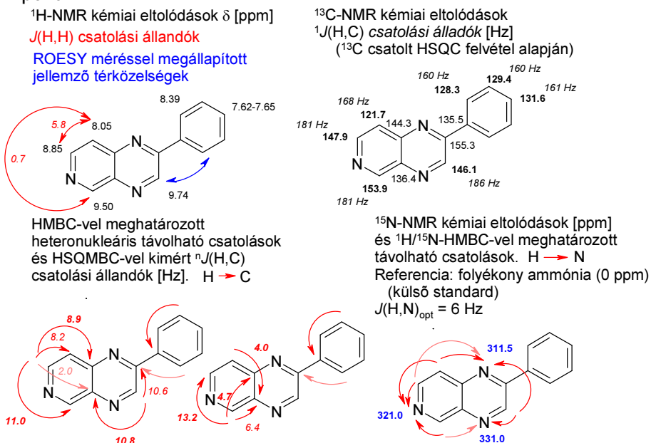
25. ábra. LA132X6 minta – pirido-pirazin származék - spektrumainak értékelése, 1 H- és 13 C-NMR jelhozzárendelés, a heteronukleáris távolható csatolási állandók, valamint az 1 H/ 15 N-HMBC spektrum értelmezése.
