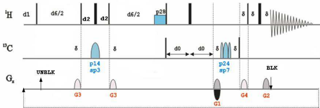
1. ábra. HSQC ed et gp jc lr nd – A Bruker pulzusprogram-könyvtárban hozzáférhető HSQMBC változat folyamatábrája. Vékony illetve vastag vonalak reprezentálják a 90 illetve 180°-os nagy kimenőteljesítményű pulzusokat. d6 = 1/2J_{lr} várakozás alatt történik meg a heteronukleáris távolható csatolások kifejlődése, ennek közepén elhelyezett G-BIRD elem szűri ki a egykötéses csatolásokat, d2 = 1/(2 \cdot J) . A mágnesezettséget INEPT pulzuspár viszi át a szénre, ott történik a második dimenzió kiépülése, majd a szén mágnesezettség refókuszálása. Inverz INEPT pulzuspár viszi vissza a mágnesezettséget a hidrogénre. G1 és G2 szelektációs gradiens pulzuspár gondoskodik a mindvégig hidrogénen volt mágnesezettség teljes defókuszálásáról.
