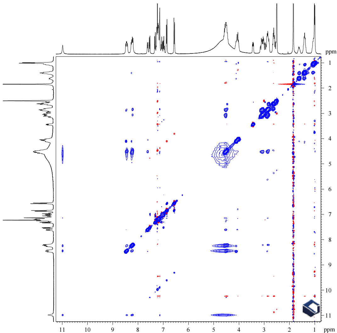
59. ábra. A TT232 minta 300 MHz-en felvett zqs-NOESY [85] spektruma
