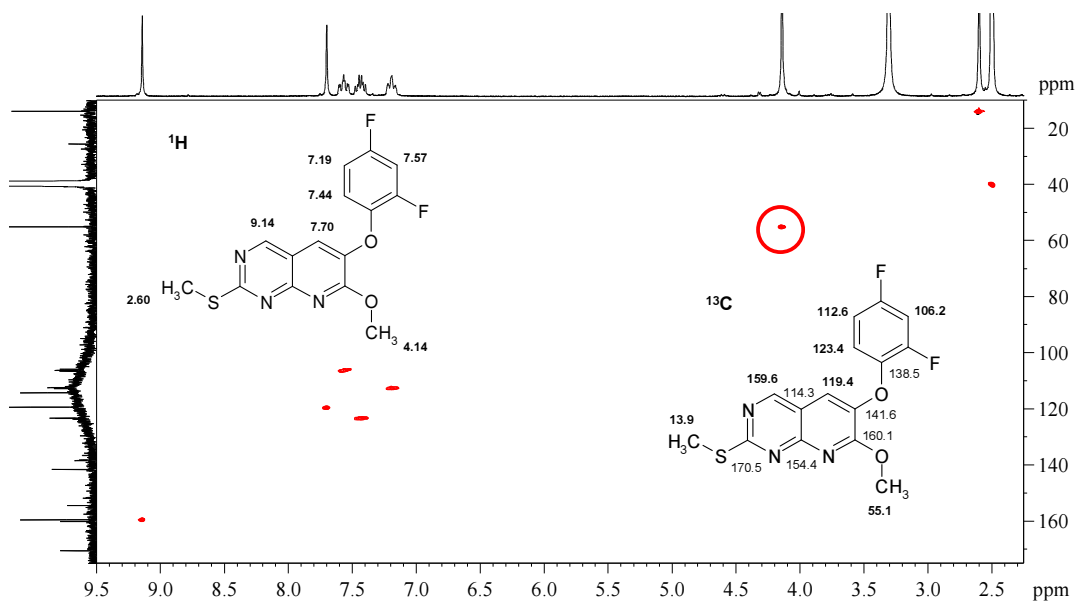
117. ábra. Izo-3 vegyület HSQC spektruma, valamint 1 H- és 13 C-NMR jelhozzárendelése. Pirossal kiemelve a szerkezet meghatározásában döntő korreláció.
