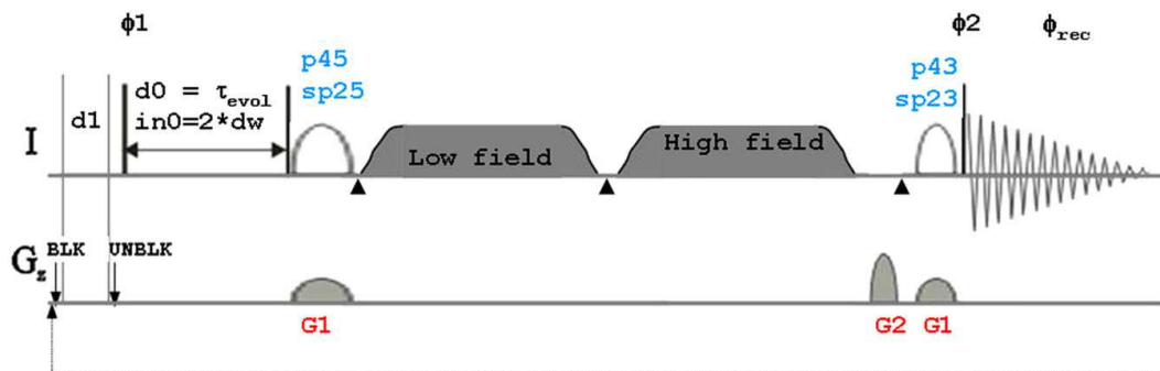
38. ábra. Az offszet-kompenzált zéró-kvantum elnyomásos adiabatikus ROESY (zqs-easy-ROESY) folyamatábrája.
