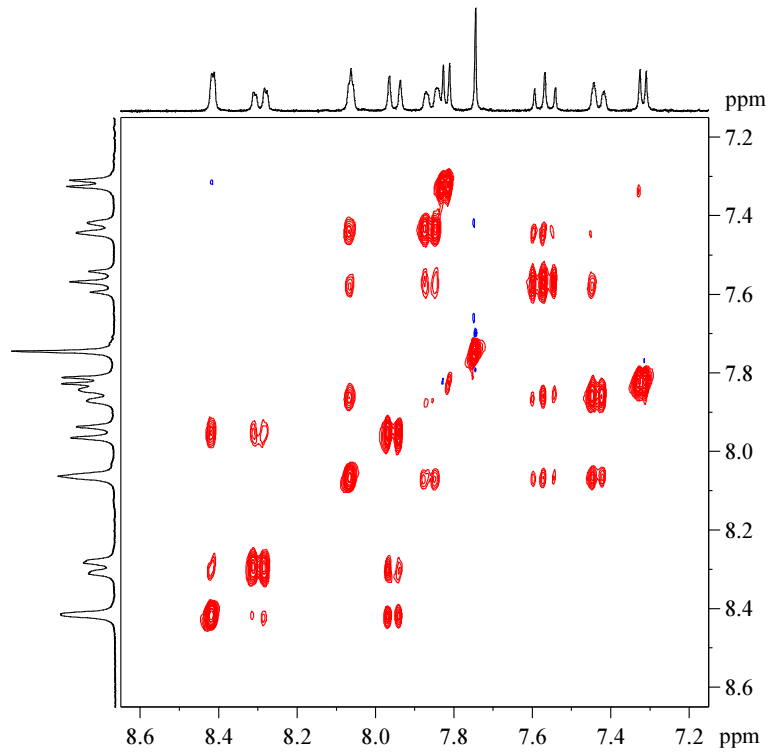
77. ábra. VIC31338 vegyület, RG1331 minta zqs-TOCSY spektruma, 2 scan * 192 kísérlet, T_{mix} = 100 msec
