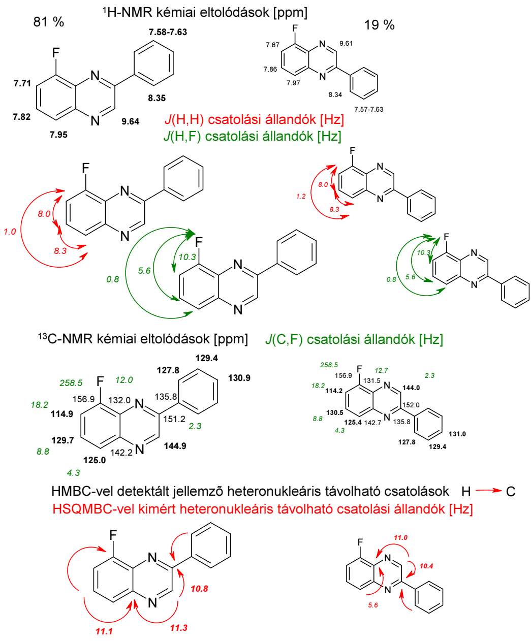
28. ábra. LA182X1 minta – két kinoxalin származék izomer keveréke - spektrumainak értékelése, 1 H- és 13 C-NMR jelhozzárendelés, a heteronukleáris távolható csatolási állandók. A mintában 19 %-os mennyiségben jelen lévő minor izomer NMR adatait is sikerült a spektrumokból kinyerni.
