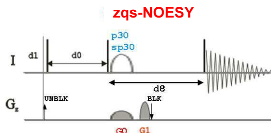
35. ábra. A zqs-NOESY módszerváltozat [85] folyamatábrája
