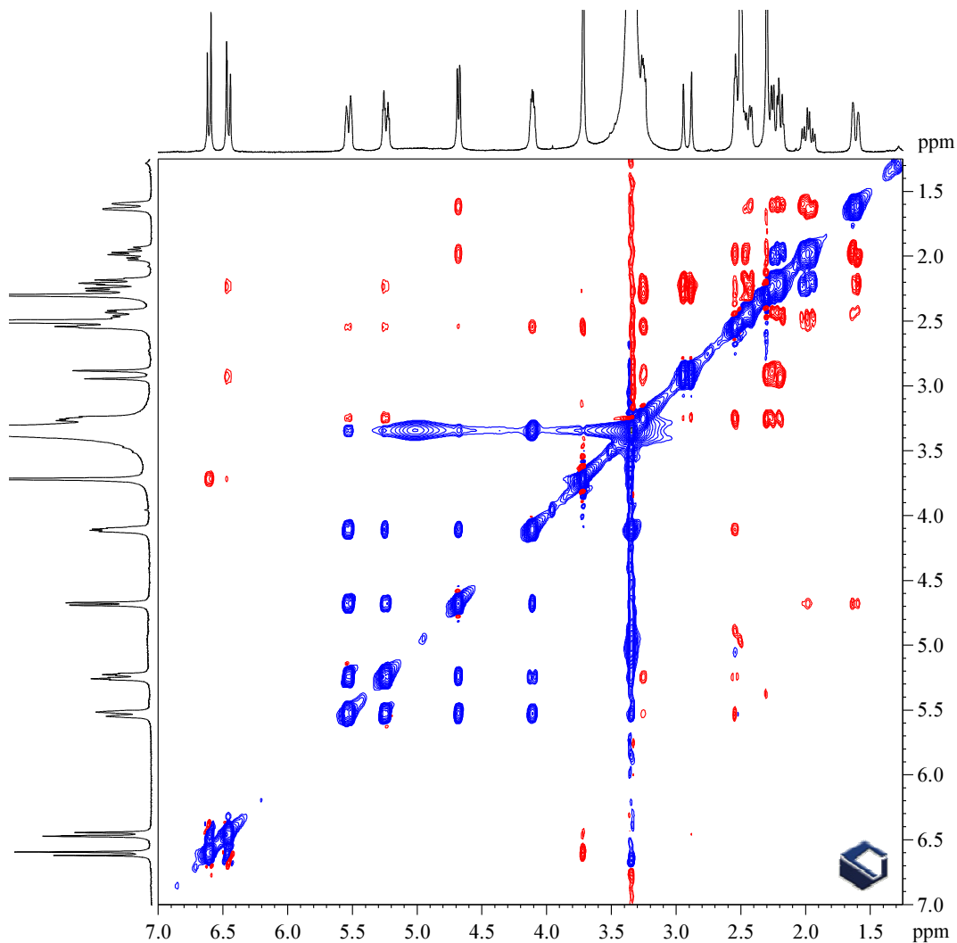
48. ábra. A kodeinnek a Bruker pulzusprogram-könyvtárban elérhető ROESYph pulzusprogrammal mért ROESY spektruma.
