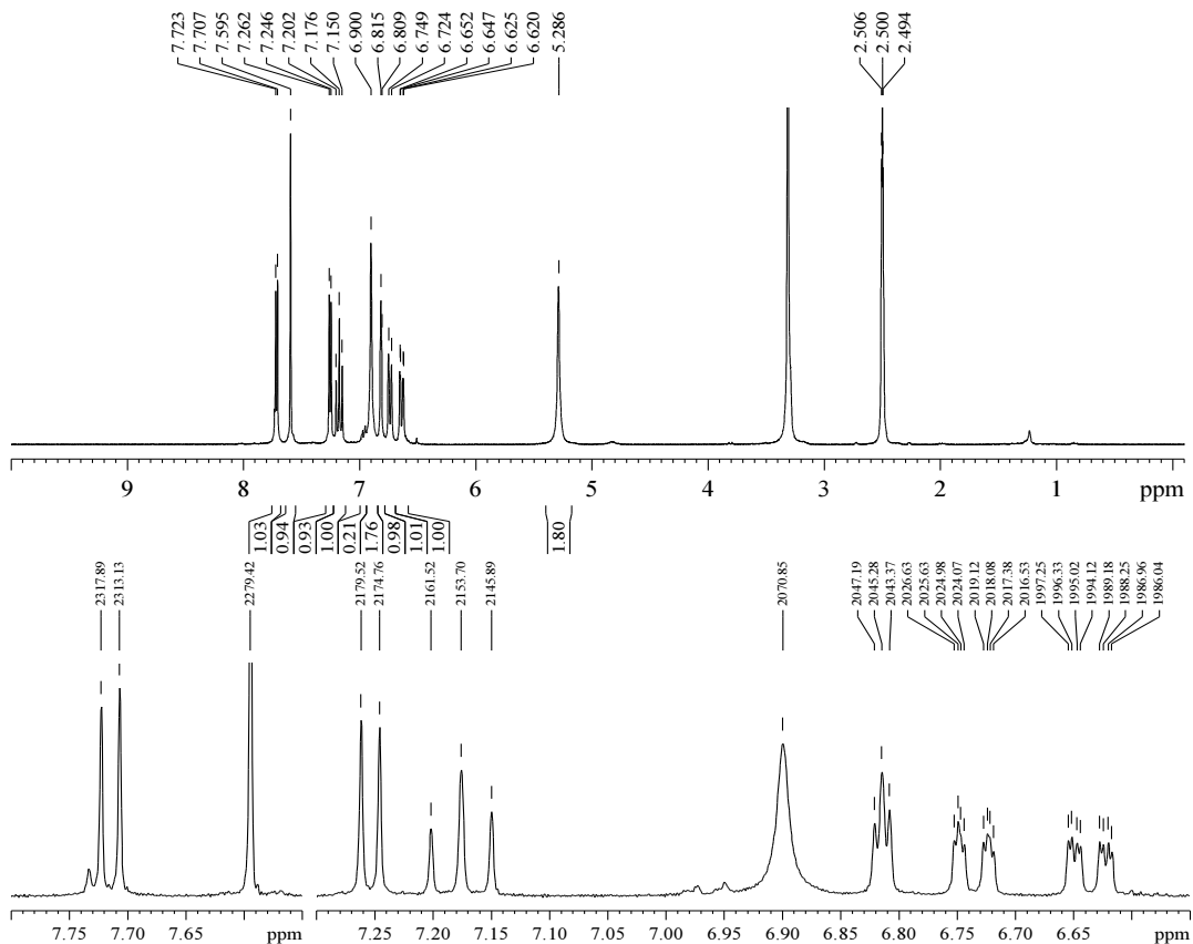
66. ábra. VIC30702 vegyület, RG-1201T minta 1 H-NMR spektruma (átnézeti és részlet)
