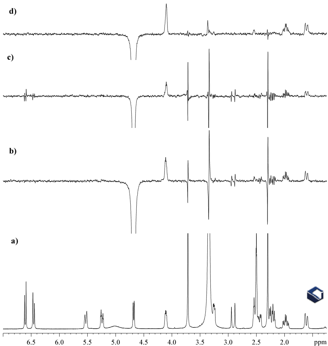
55. ábra. A kodein válogatott szelektív 1D spektrumai.
